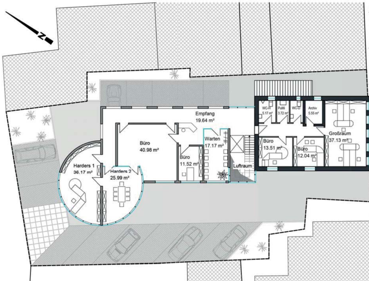
OBERGESCHOSS M 1:200
